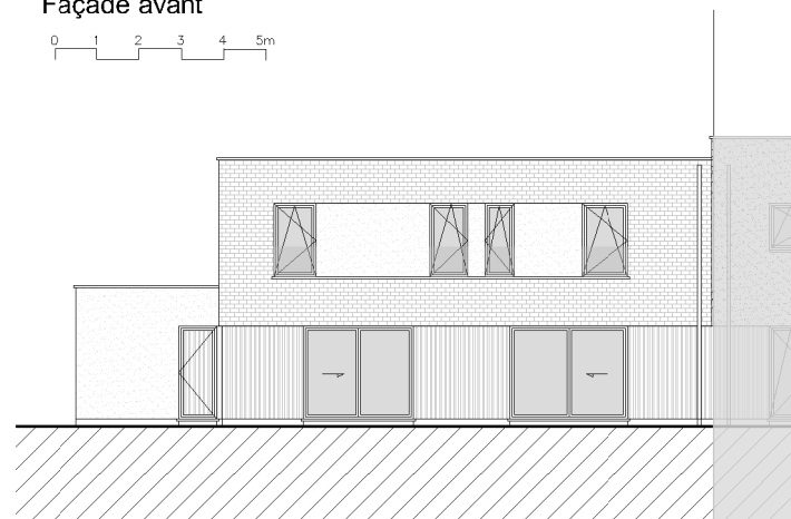
Façade avant
