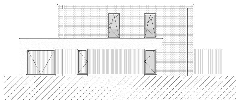
Façade avant
