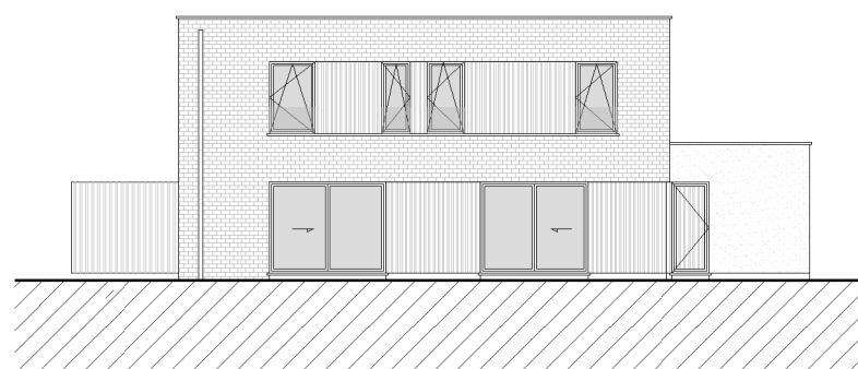
Façade arrière
