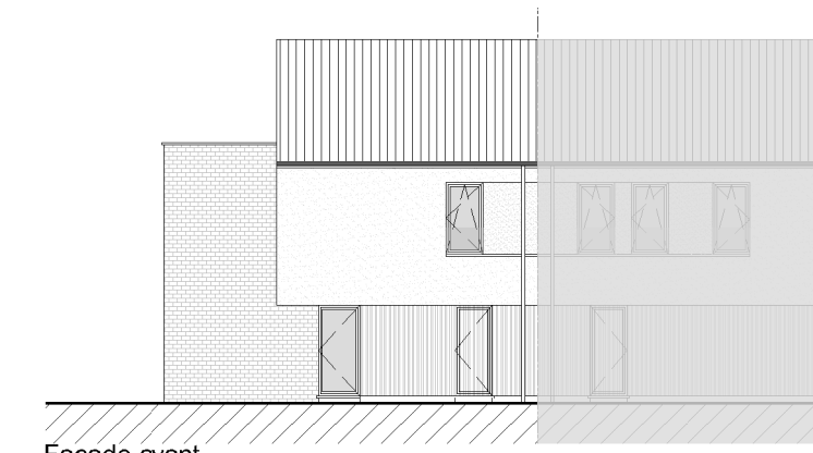
Façade avant
